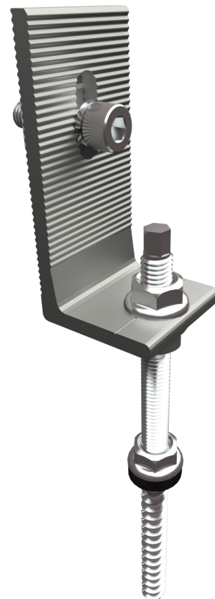
Кронштейн кріплення для металочерепиці з метизами
