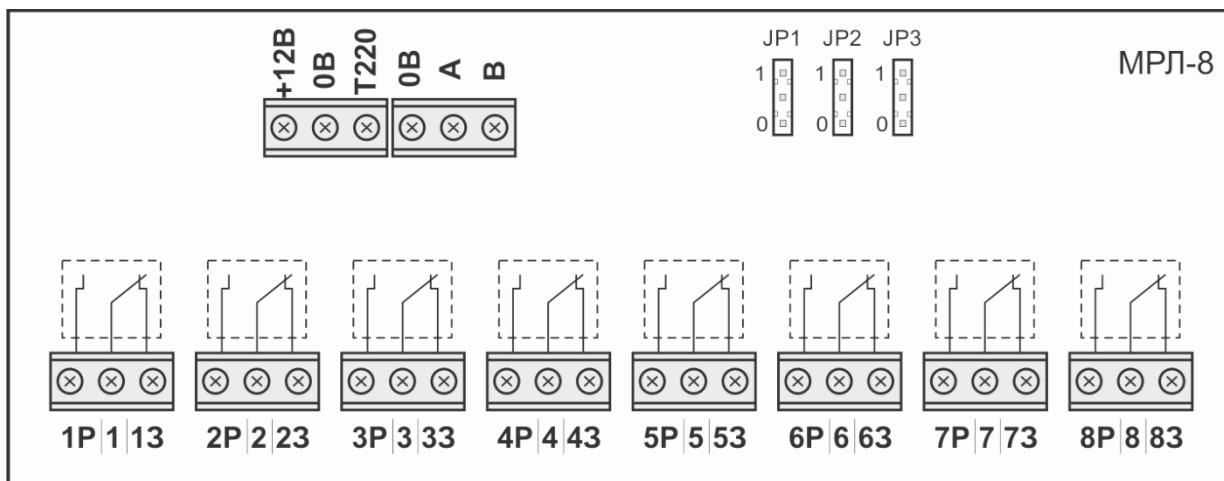
Рисунок 7.9 – Підключення входів та виходів МРЛ-8 Призначення клем МРЛ-8 наведено в таблиці 7.4.
