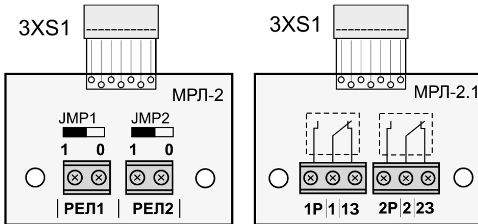
Рисунок 7.8 – Модулі МРЛ
